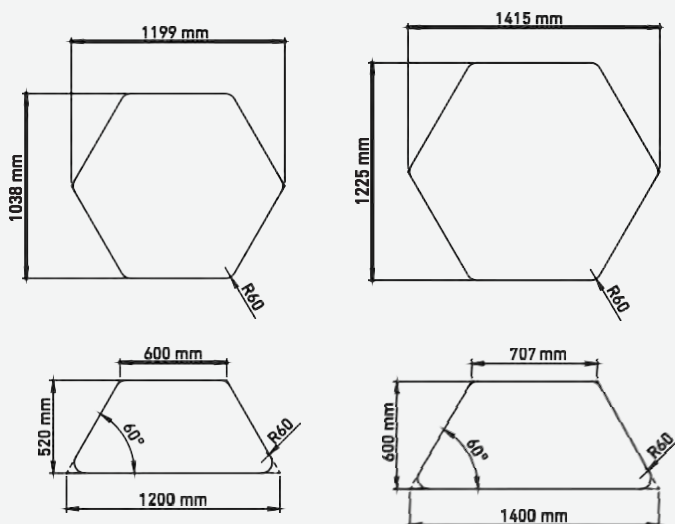
Schițe cu dimensiuni
