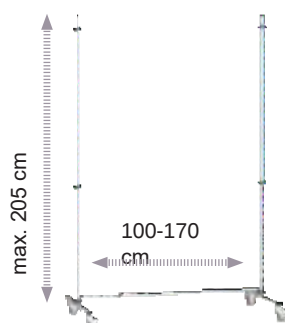
T-ÁLV-G Stativ T cu roți
